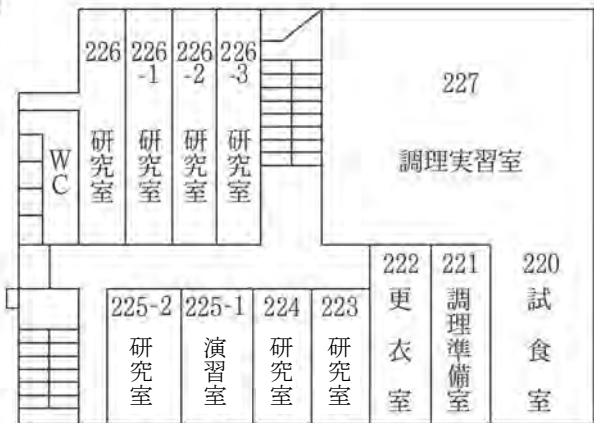
【 2 階】
